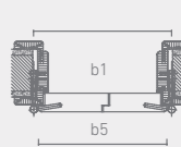
Coupe horizontale du revêtement (RF) 2 vantaux, à feuillure
