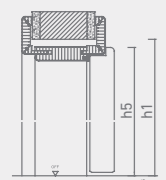
Vertikalschnitt Zarge mit Rundkante
