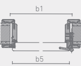
Horizontalschnitt Zarge mit Rundkante 1-flügelig gefälzte Türen
