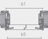
Horizontalschnitt Zarge mit Rundkante 2-flügelig gefälzte Türen
