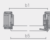
Coupe horizontale du revêtement (RF) 1 vantail, à feuillure
