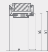
Coupe verticale du revêtement (RF)
