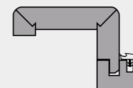
4 ZARGE MIT RUNDKANTE CADRE AVEC CHANT ARRONDIS
